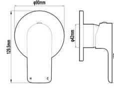
BASSINI WALL MIXER CODE 82810, 82810-B, 82810-BC, 82810-BG, 82810-BR, 82810-GM, 82810-RG, 82810-W
