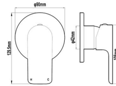
BASSINI WALL MIXER CODE 82810, 82810-B, 82810-BC, 82810-BG, 82810-BR, 82810-GM 82810-RG, 82810-W
