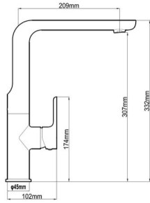
BASSINI SINK MIXER CODE 82800, 82800-B, 82800-BC, 82800-BG, 82800-BR, 82800-GM 82800-RG, 82800-W
