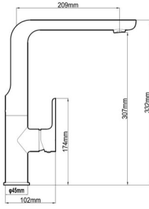
BASSINI SINK MIXER CODE 82800, 82800-B, 82800-BC, 82800-BG, 82800-BR, 82800-GM, 82800-RG, 82800-W
